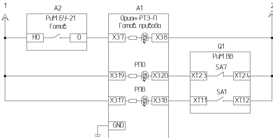
Рисунок Б 4 – Схема подключения БУ к Орион РТЗ. Токовые цепи. Цепи питания. Оперативные цепи
