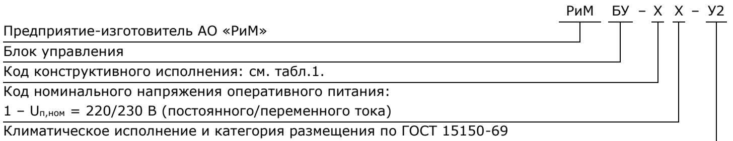
Рисунок 1 – Структура условного обозначения БУ
