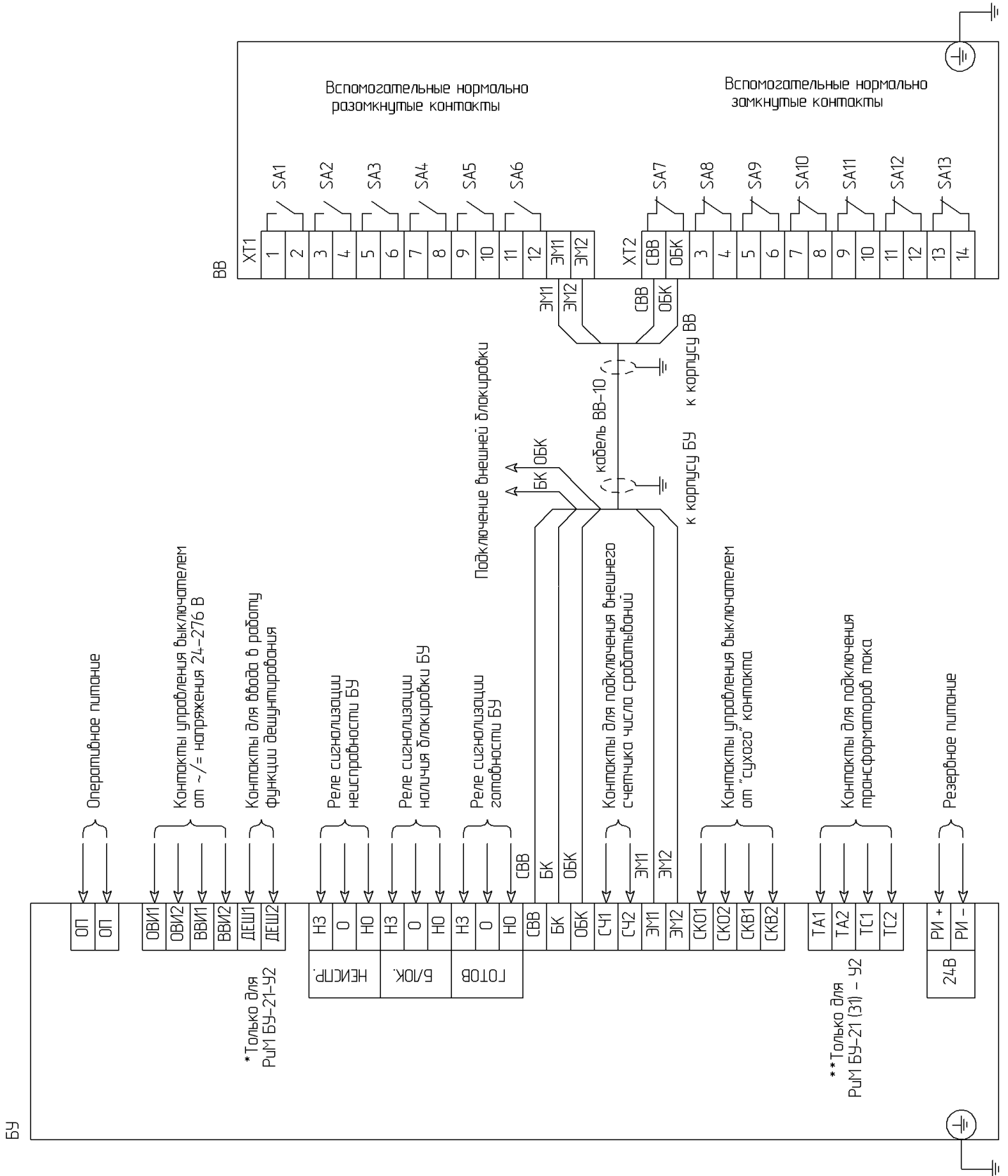
Рисунок Б 1 – Схема подключения БУ к ВВ
