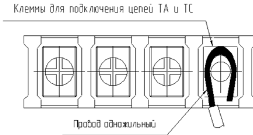
Рисунок 11 – Укладка одножильного провода
