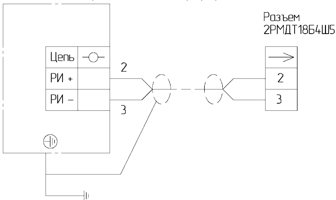
Рисунок В 1 - Подключение разъема 2РМДТ18Б4Ш5 к БУ серии 51
