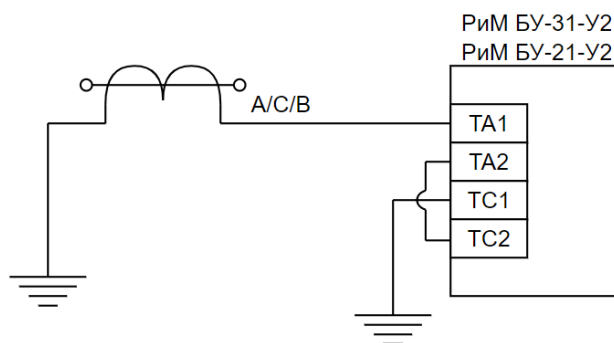
Рисунок 7 – Однофазная (двухфазная) схема подключения БУ серий 21, 31 к ТТ
