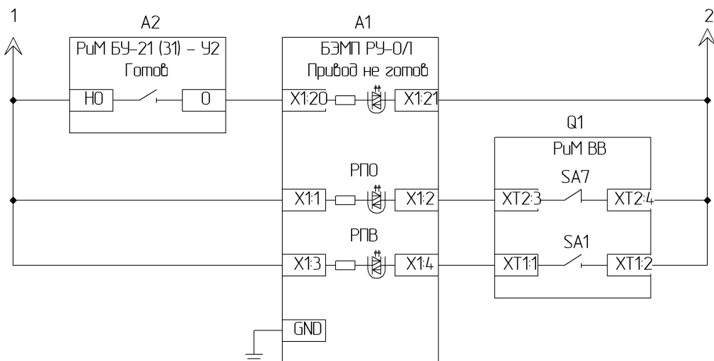
Рисунок Б 2 – Схема подключения БУ к БЗМП РУ. Токовые цепи. Цепи питания. Оперативные цепи
