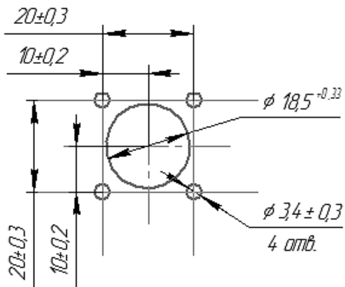
Рисунок В 2 - Разметка отверстий для монтажа разъема 2РМДТ18Б4Ш5
