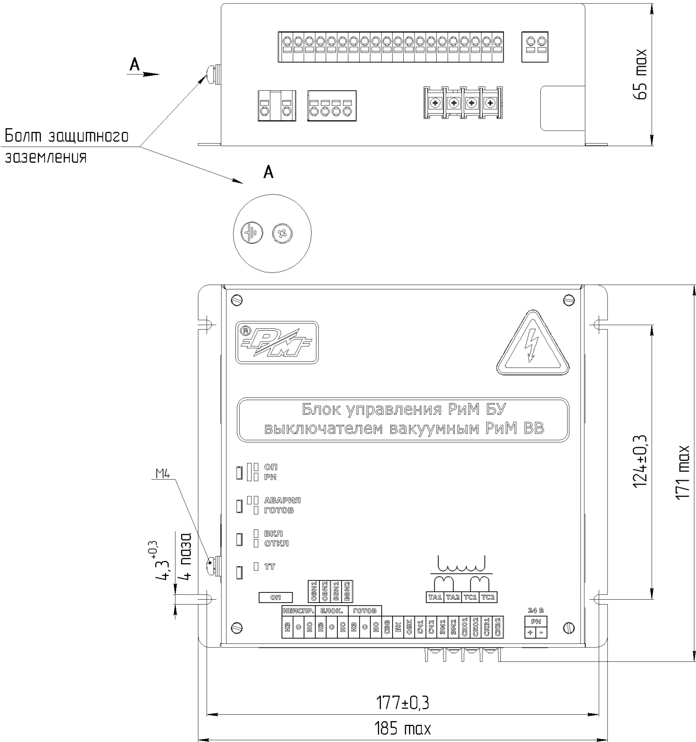
Рисунок А 2 - Габаритные установочные и присоединительные размеры РИМ БУ – 31 – У2
