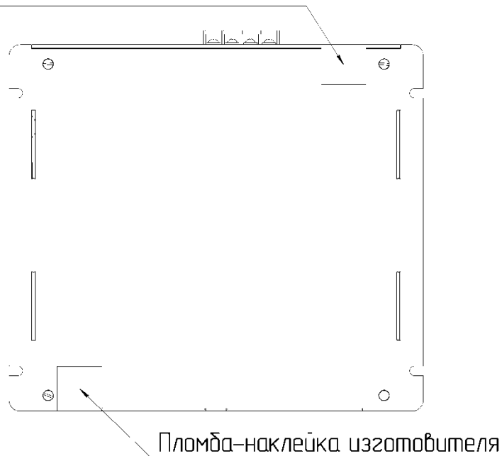
Рисунок 10 – Схема пломбирования БУ
