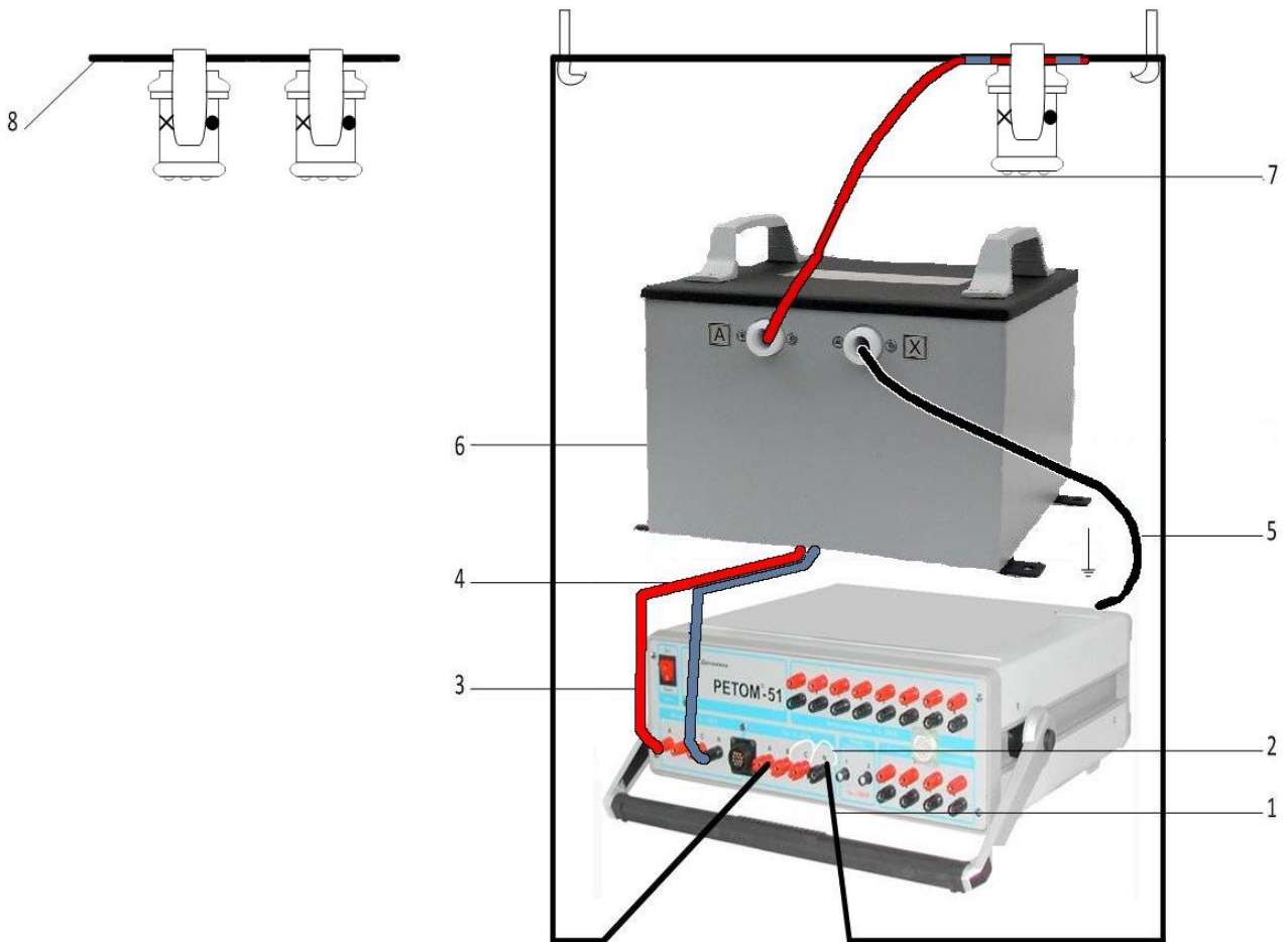
Рисунок 2.3 – Порядок установки
