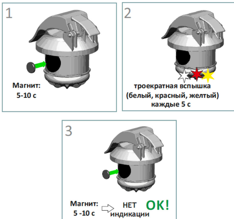
Рисунок 8 – Тестирование индикатора ИКЗ-В54Л-УЗ
