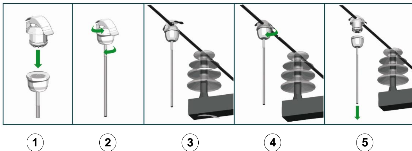
Рисунок 16 – Порядок установки индикатора ИКЗ-В54Л без отключения подачи напряжения
