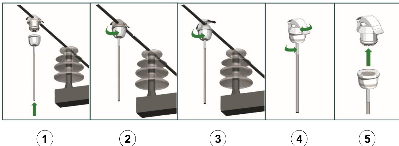
Рисунок 17 – Порядок демонтажа индикатора ИКЗ-В54Л без отключения подачи напряжения
