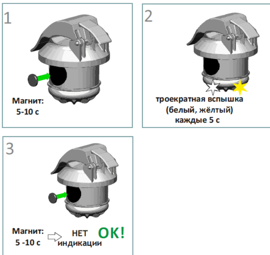
Рисунок 15 – Тестирование индикатора ИКЗ-В52Л
