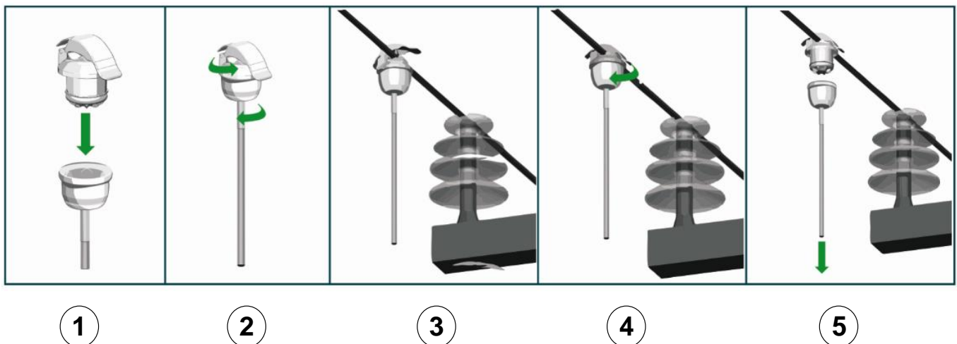
Рисунок 20 – Порядок установки индикатора ИКЗ-В52Л без отключения подачи напряжения
