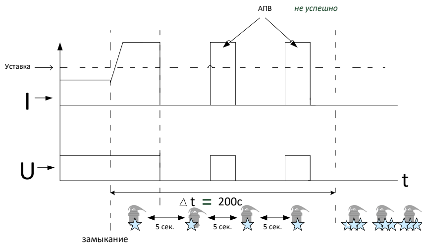
Рисунок 6 – Работа ИКЗ-В52Л при устойчивом замыкании
