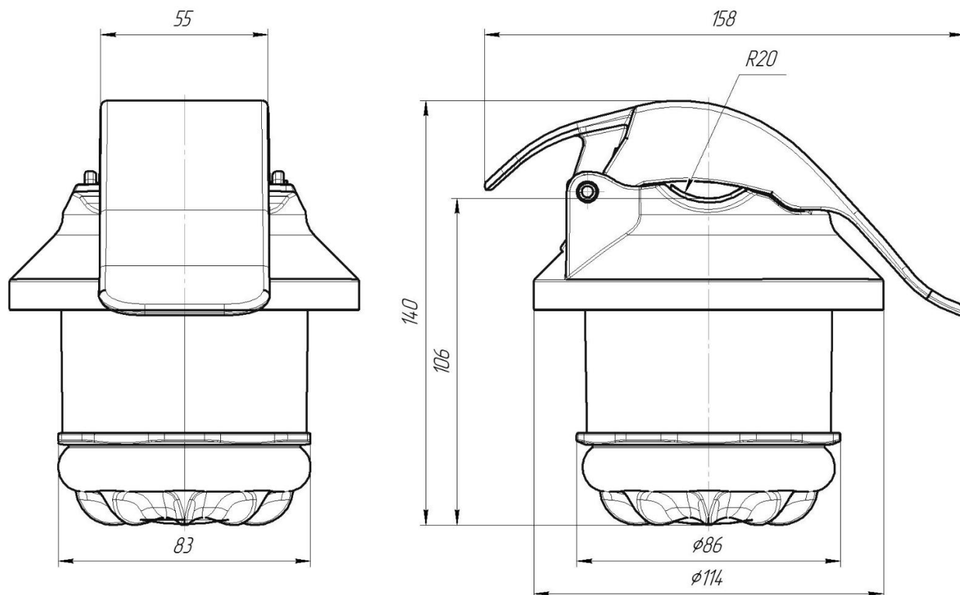
Рисунок 1.2 – Габаритные размеры ИКЗ-В52Л-С
