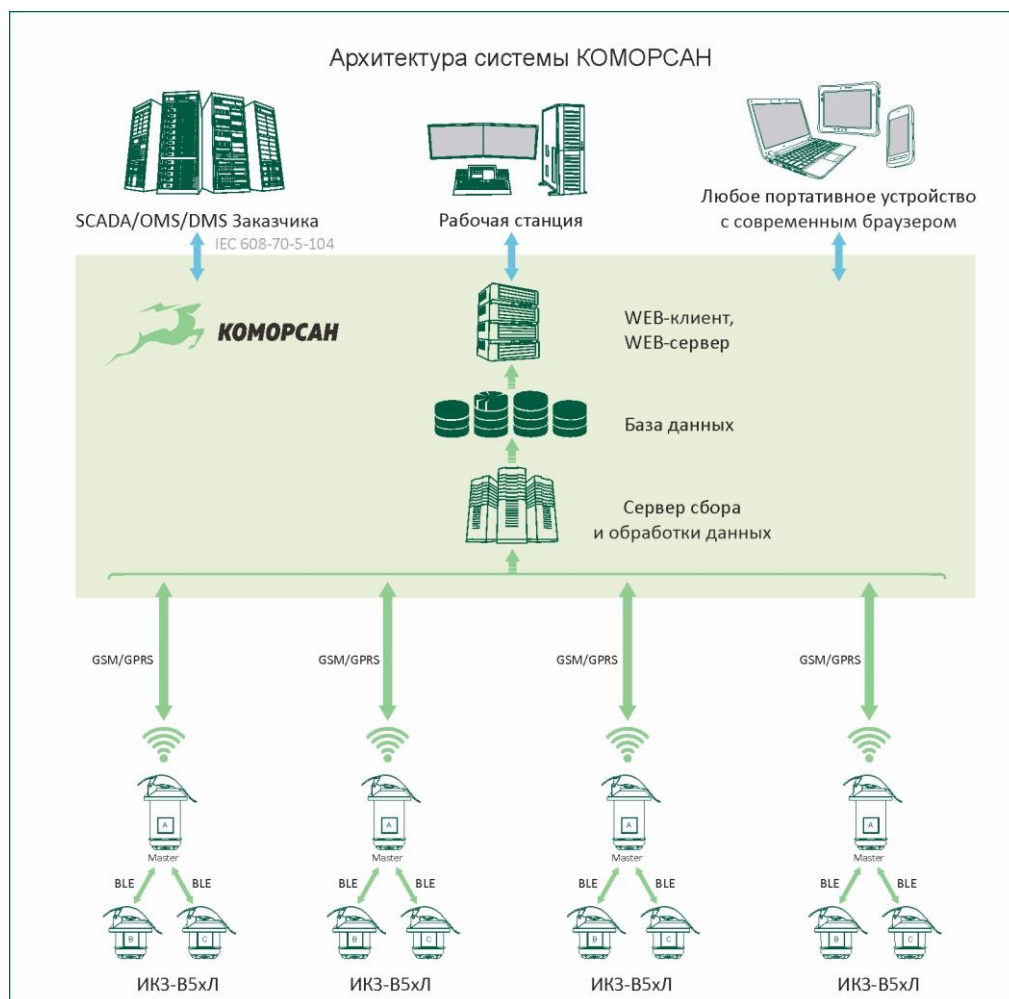
Рисунок 3 – Схема функциональной структуры мониторинга линий электропередачи
