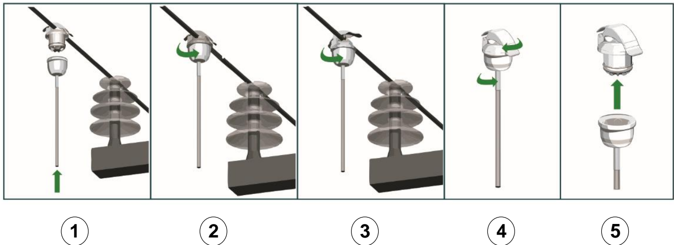
Рисунок 21 – Порядок демонтажа индикатора ИКЗ-В52Л без отключения подачи напряжения
