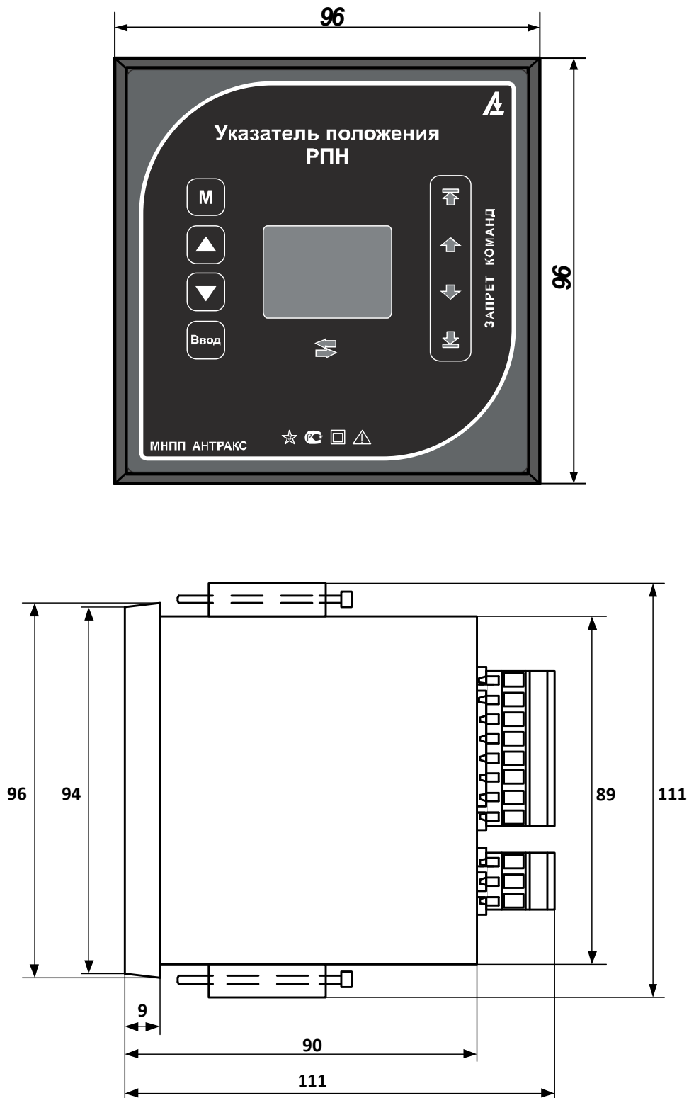
Рис. 1.1 Габаритные размеры указателя положения РПН УП 25-Г (щитовой вариант).
