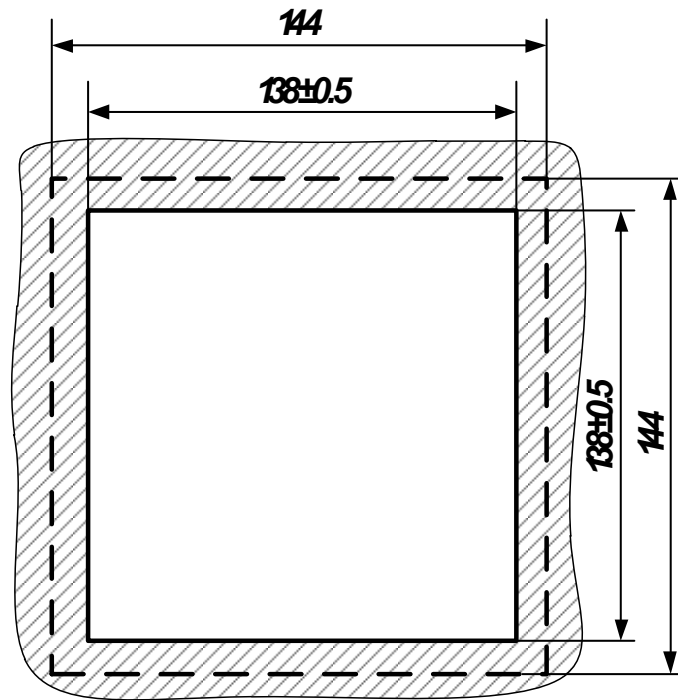
Рис. 2.1 Размеры вырубного отверстия в щите для установки указателя положения УП 25-Б
