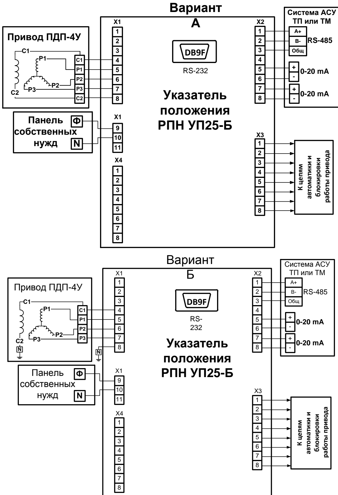
Рис. 4.1 Схемы привязки УП 25-Б-2ТП-3 к приводу типа ПДП-4У
