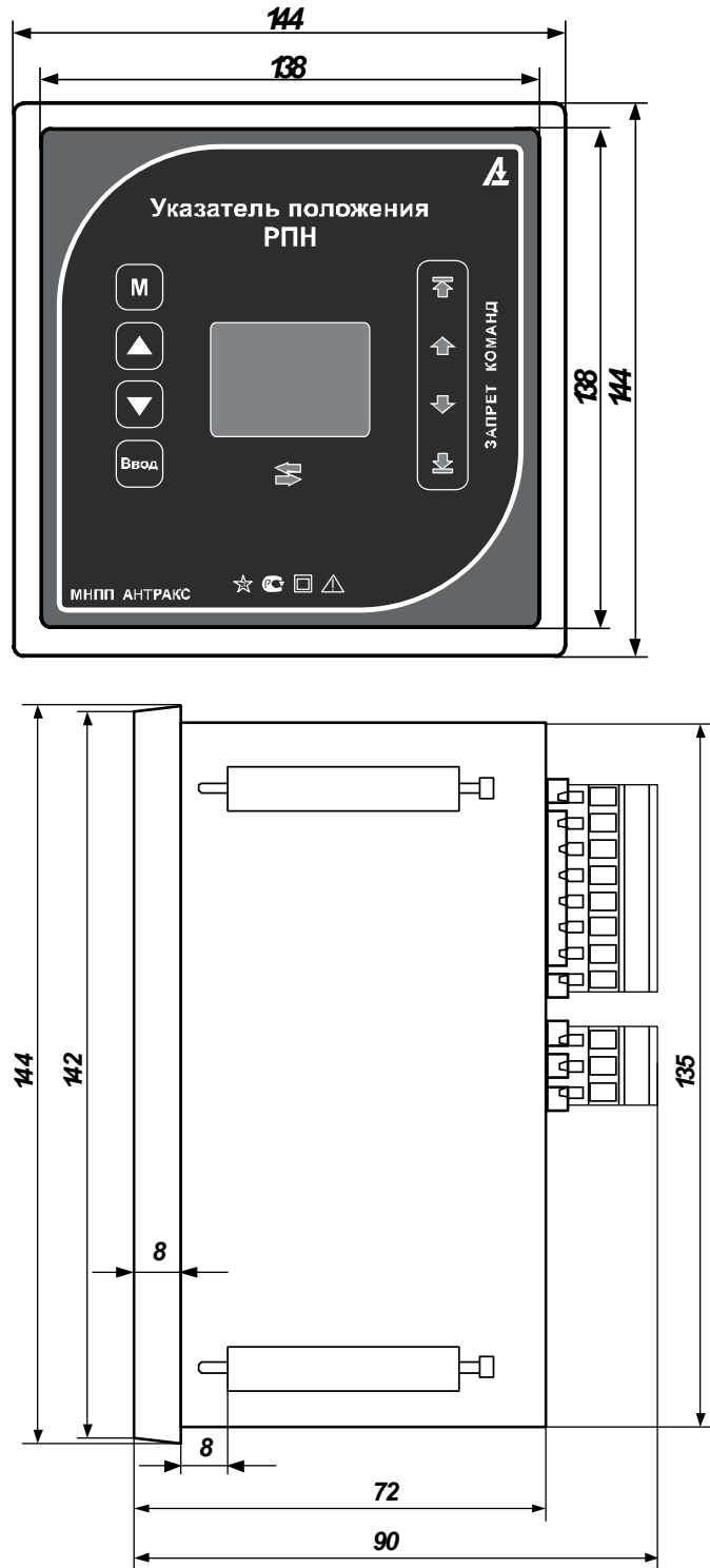
Рис. 1.1 Габаритные размеры указателя положения РПН УП 25-Б (щитовой вариант).
