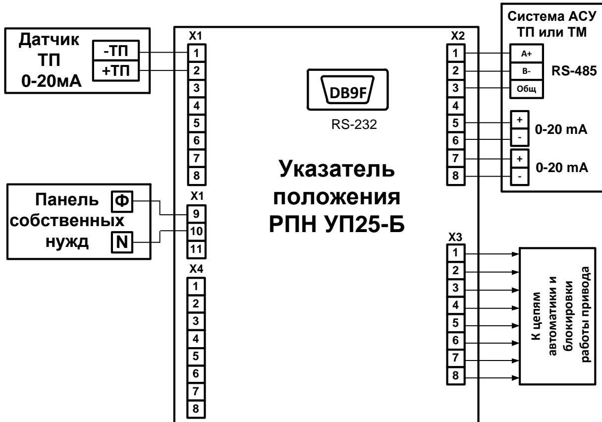
Рис. 4.3 Схема привязки УП 25-Б-2ТП-3 к датчику «Токовая петля» 0-20 мА
