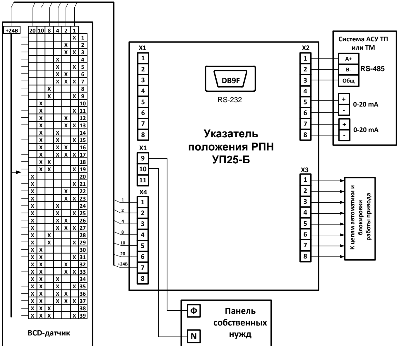
Рис. 4.4 Схема привязки УП 25-Б-2ТП-3 к BCD-датчику
