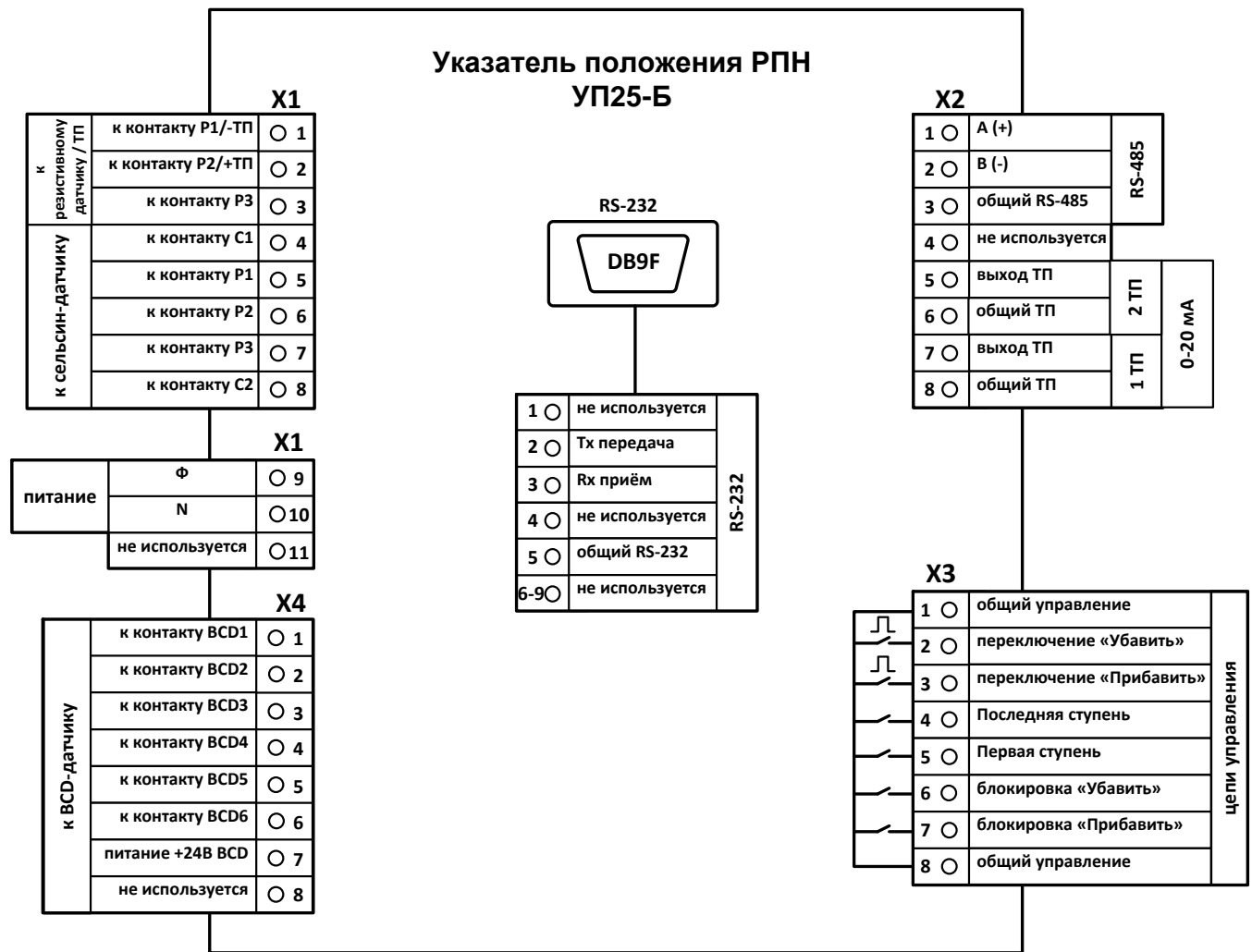
Рис. 3.1 Схема подключения УП 25-Б-2ТП-3
