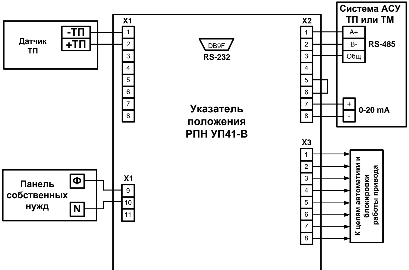
Рис. 4.1 Схема привязки УП 41-В к приводу.
