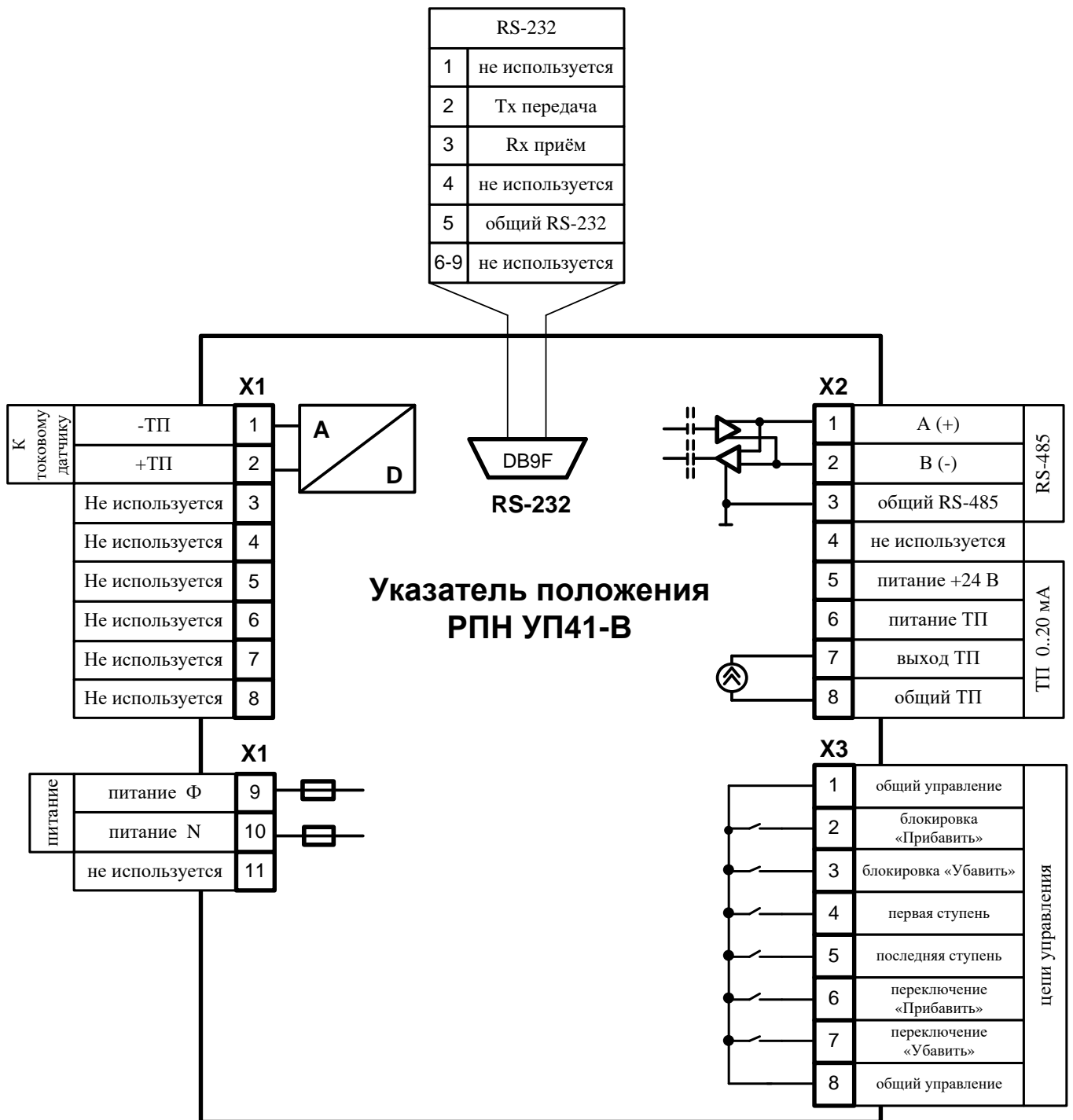
Рис. 3.1 Схема подключения УП 41-В
