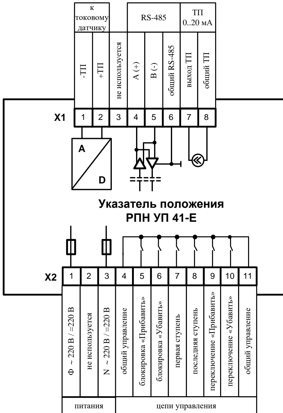
Рис. 3.1 Схема подключения УП 41-Е
