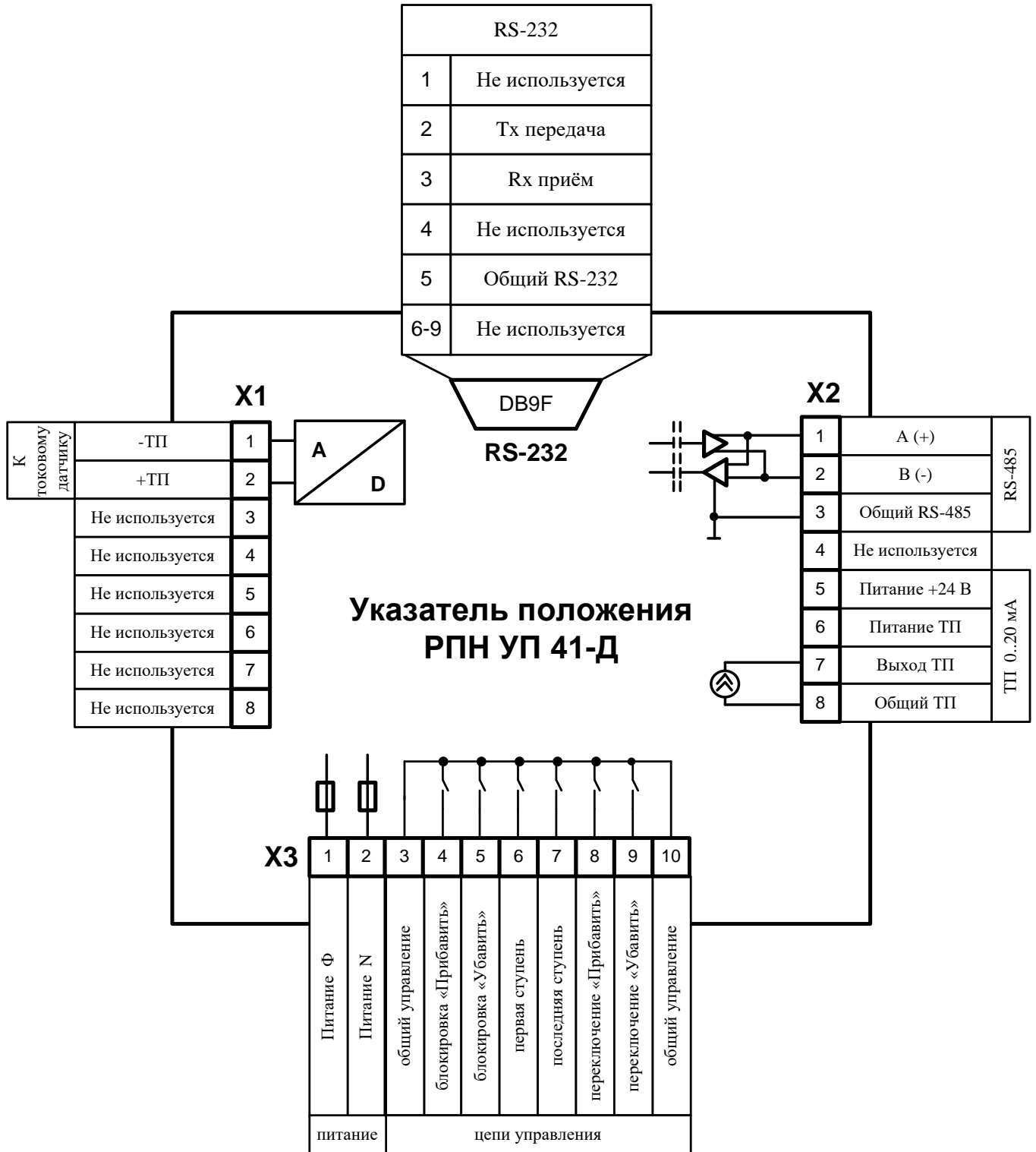
Рис. 3.1 Схема подключения УП 41-Д
