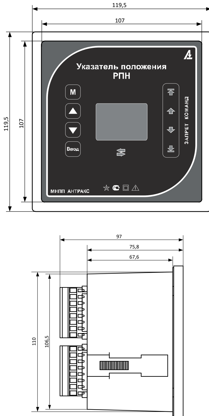
Рис. 1.1 Габаритные размеры щитового варианта указателя положения РПН УП 41-Д
