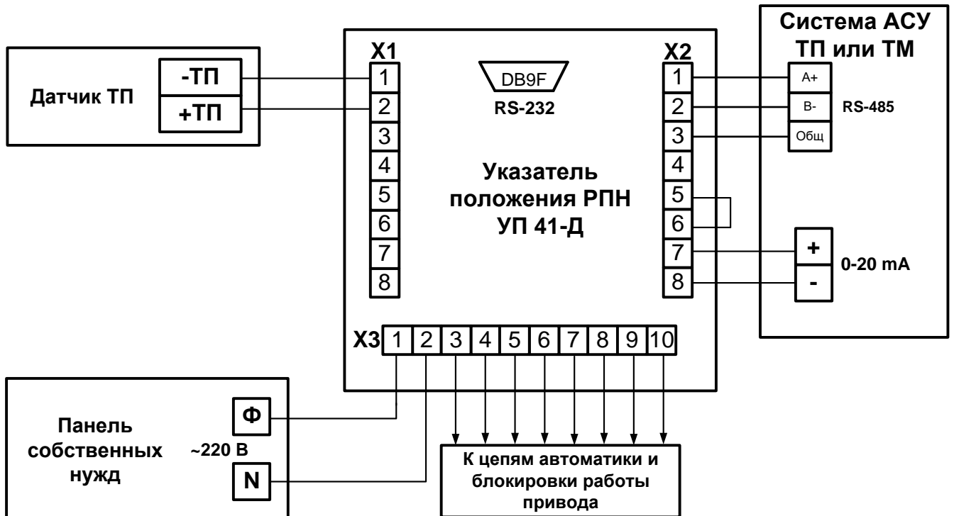
Рис. 4.1 Схема привязки УП 41-Д к приводу типа MR.
