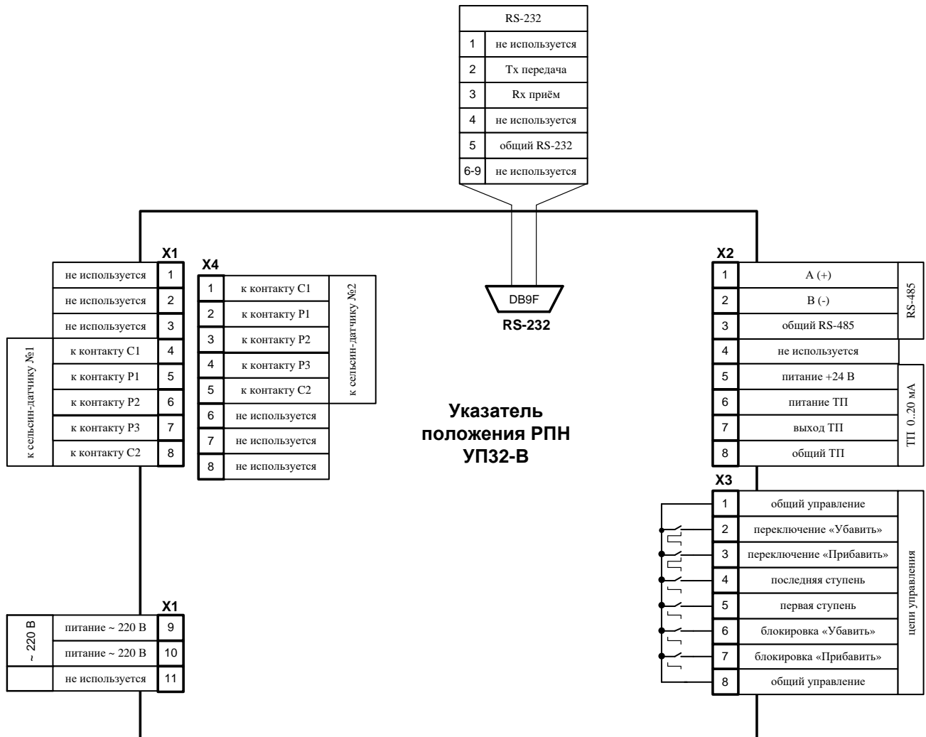
Рис. 3.1 Схема подключения УП 32-В
