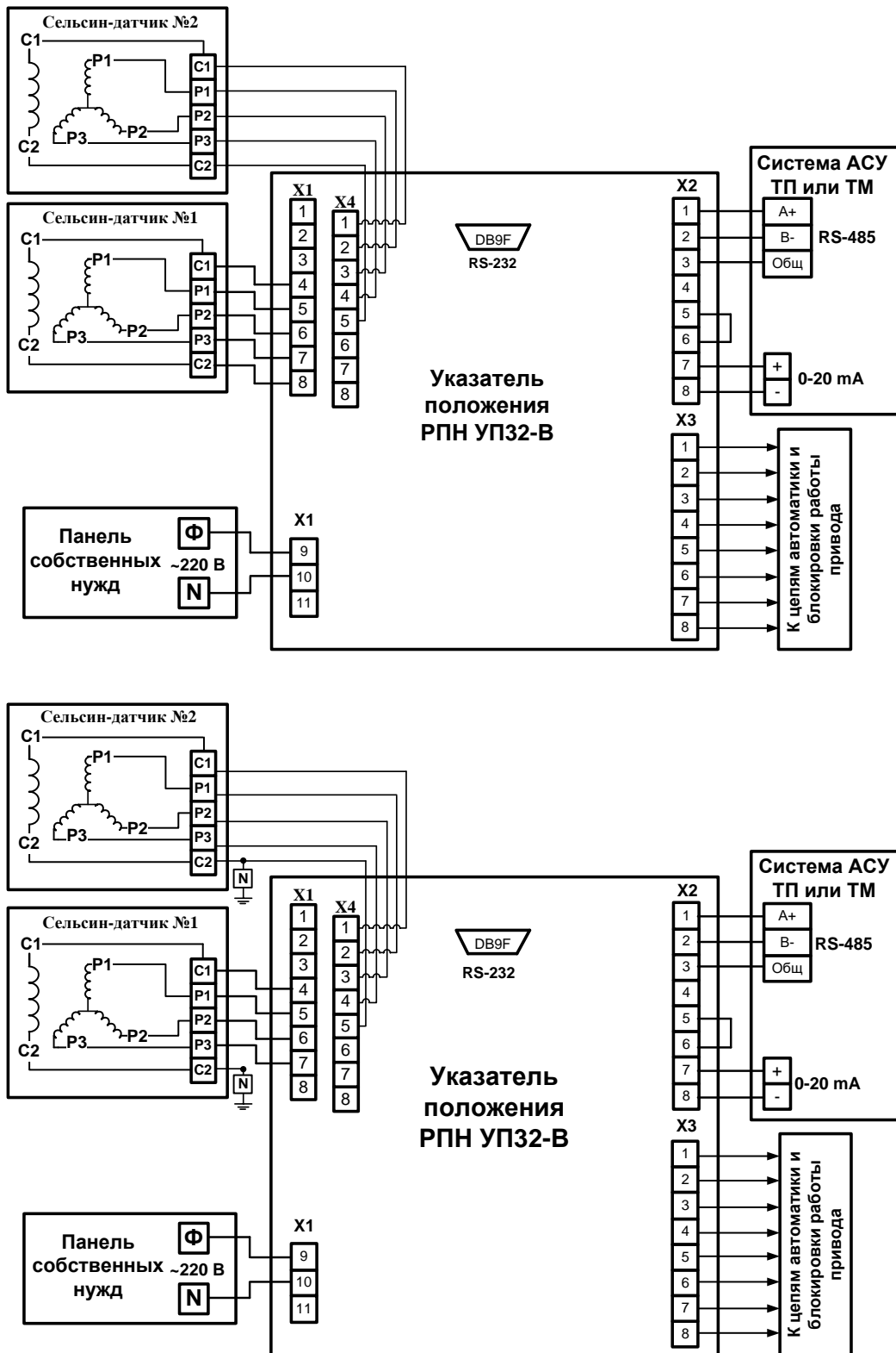
Рис. 4.1 Схемы привязки УП 32-В к приводу типа ПДП-4У
