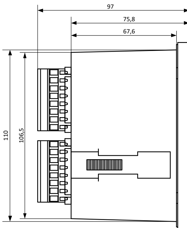
Рис. 1.1 Габаритные размеры настенного варианта указателя положения РПН УП 32-В
