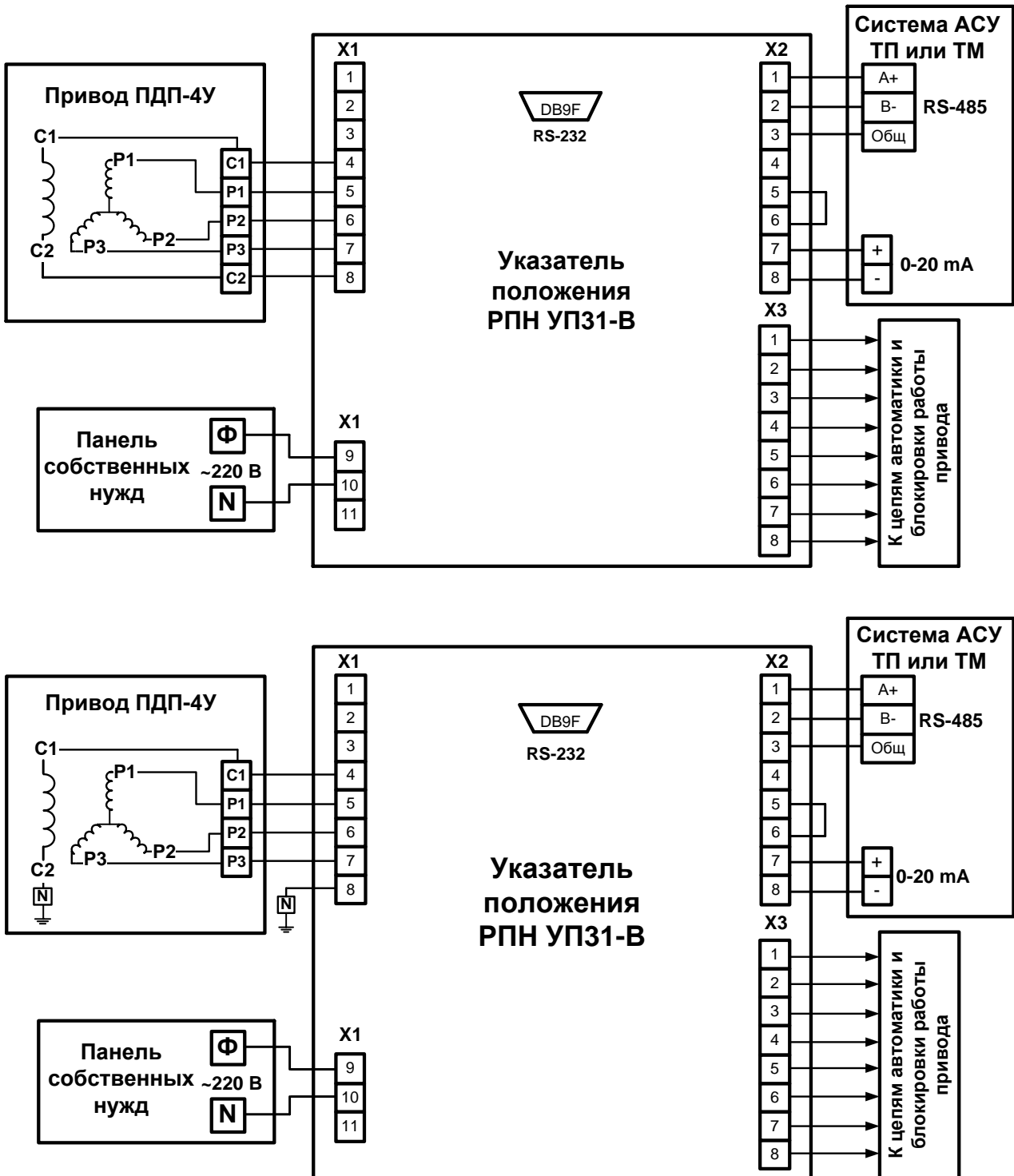
Рис. 4.1 Схемы привязки УП 31-В к приводу типа ПДП-4У
