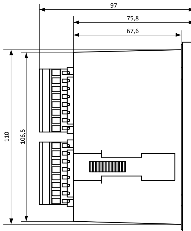
Рис. 1.1 Габаритные размеры настенного варианта указателя положения РПН УП 31-В
