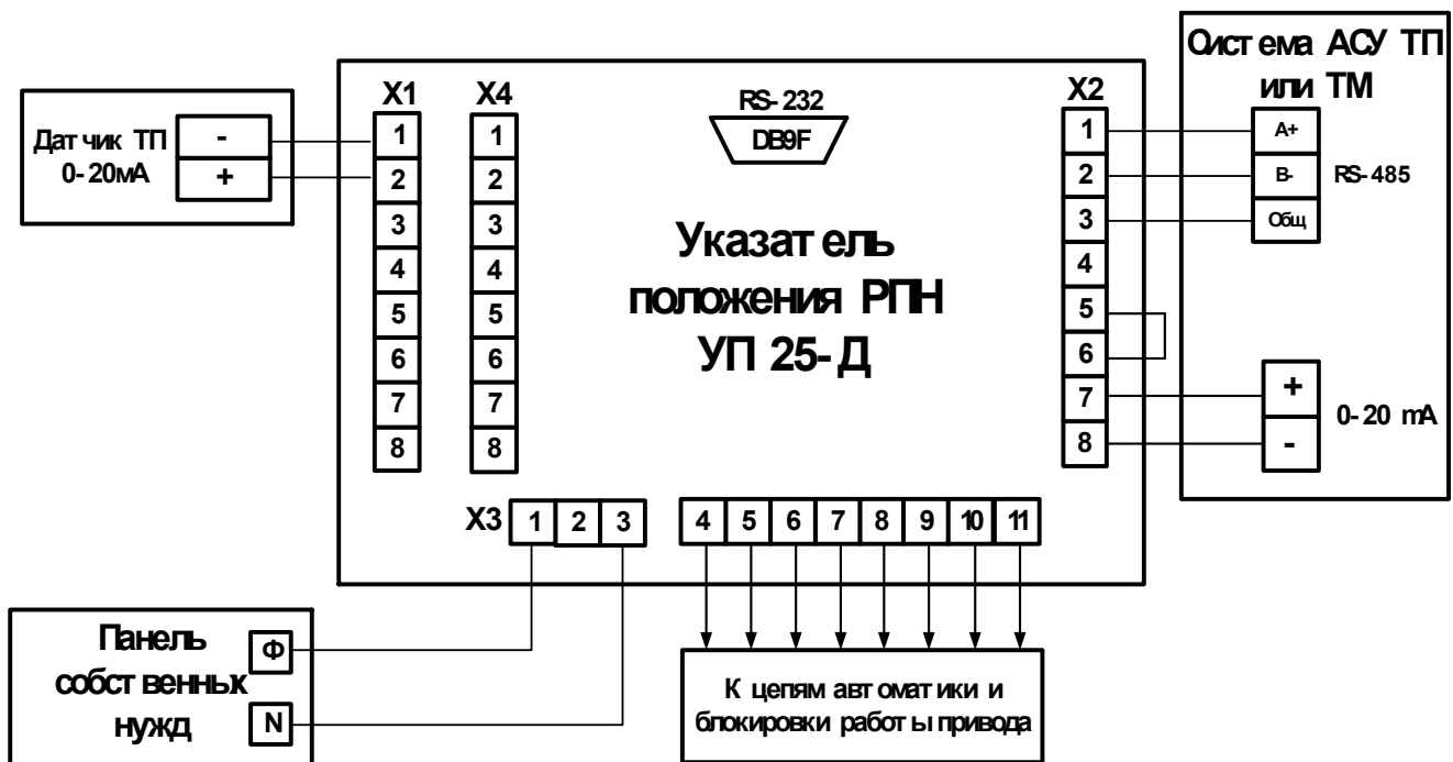
Рис. 4.3 Схема привязки УП 25-Д к датчику «Токовая петля» 0-20 мА.
