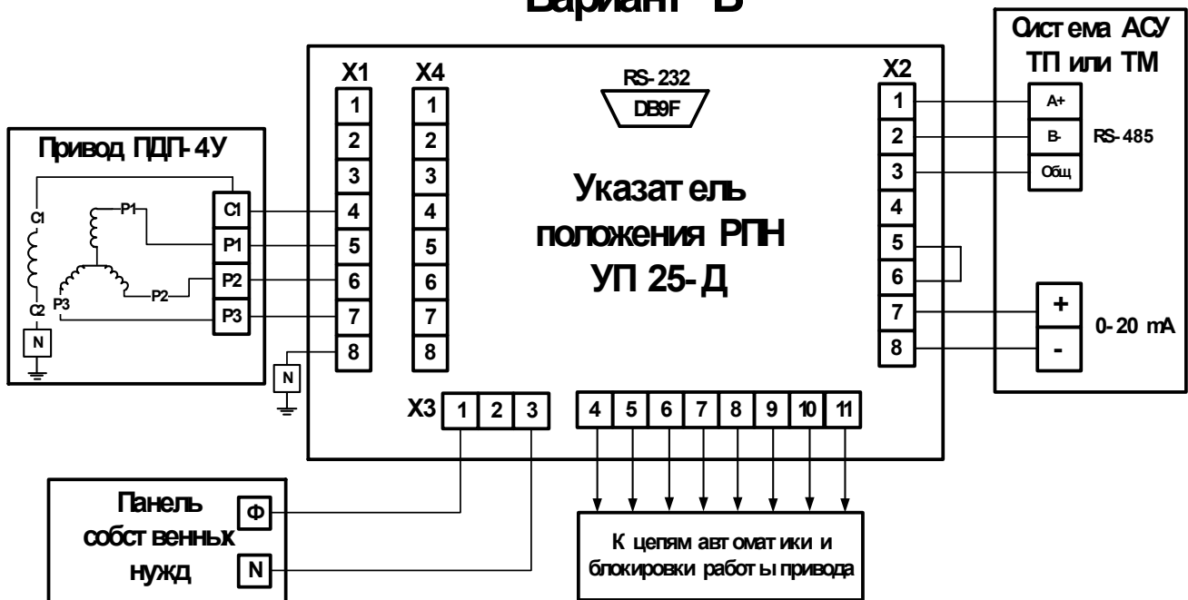
Рис. 4.1 Схемы привязки УП 25-Д к приводу типа ПДП-4У.
