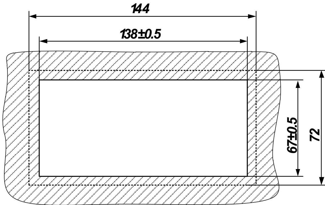
Рис. 2.1 Размеры вырубного отверстия в щите для установки указателя положения УП 25-Д.
