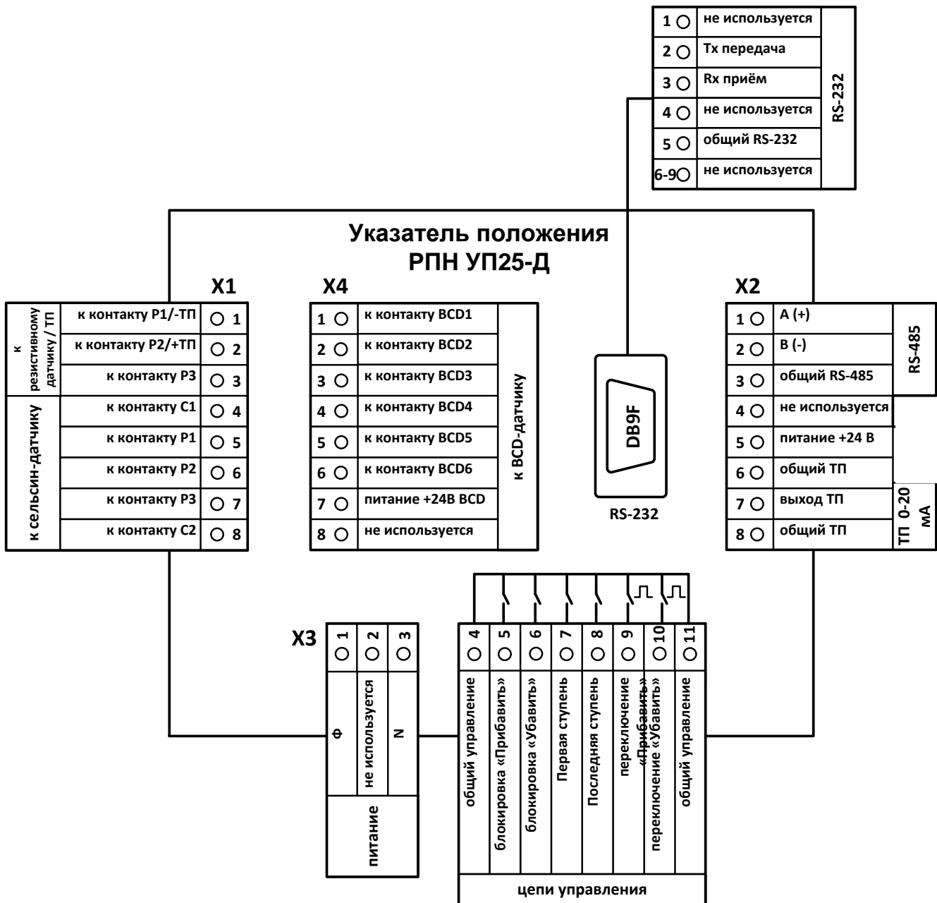
Рис. 3 Схема подключения УП 25-Д.
