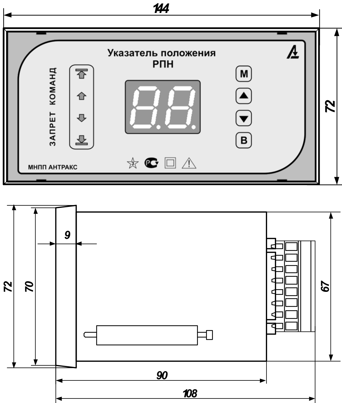
Рис. 1.1 Габаритные размеры указателя положения РПН УП 25-Д (щитовой вариант).
