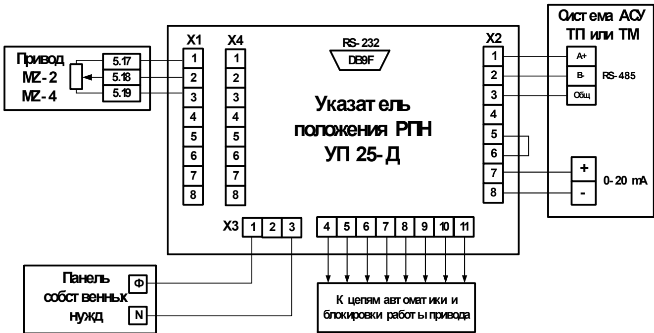
Рис. 4.2 Схема привязки УП 25-Д к приводу типа MZ-2, MZ-4.
