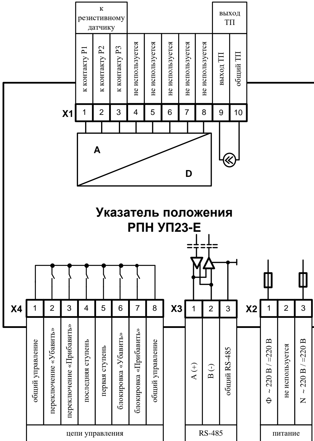
Рис. 3.1 Схема подключения УП 23-Е
