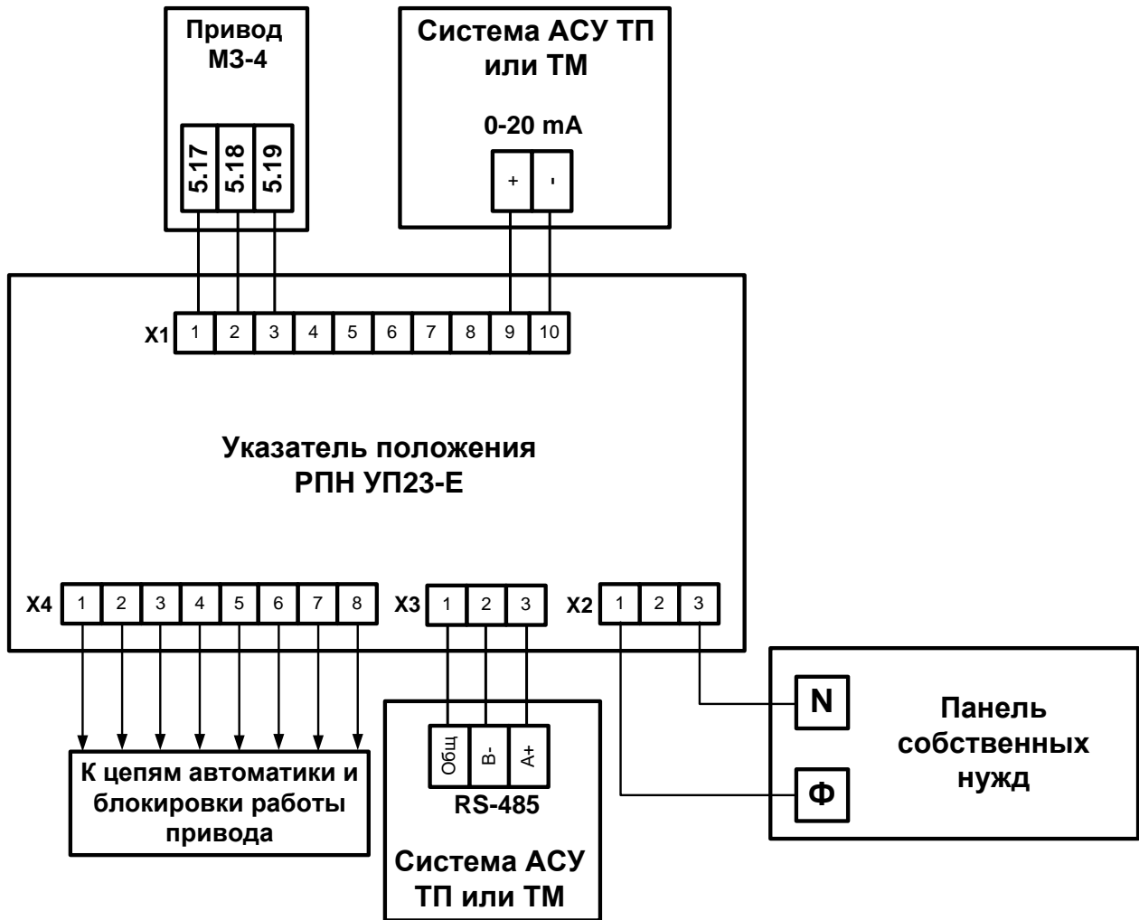
Рис. 4.1 Схема привязки УП 23-Е к приводу.
