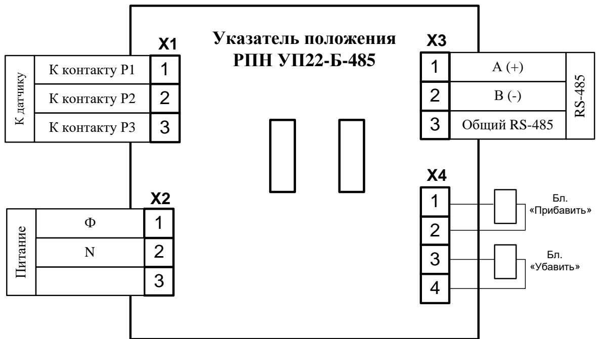
Рис. 3.1 Схема подключения УП 22-Б
