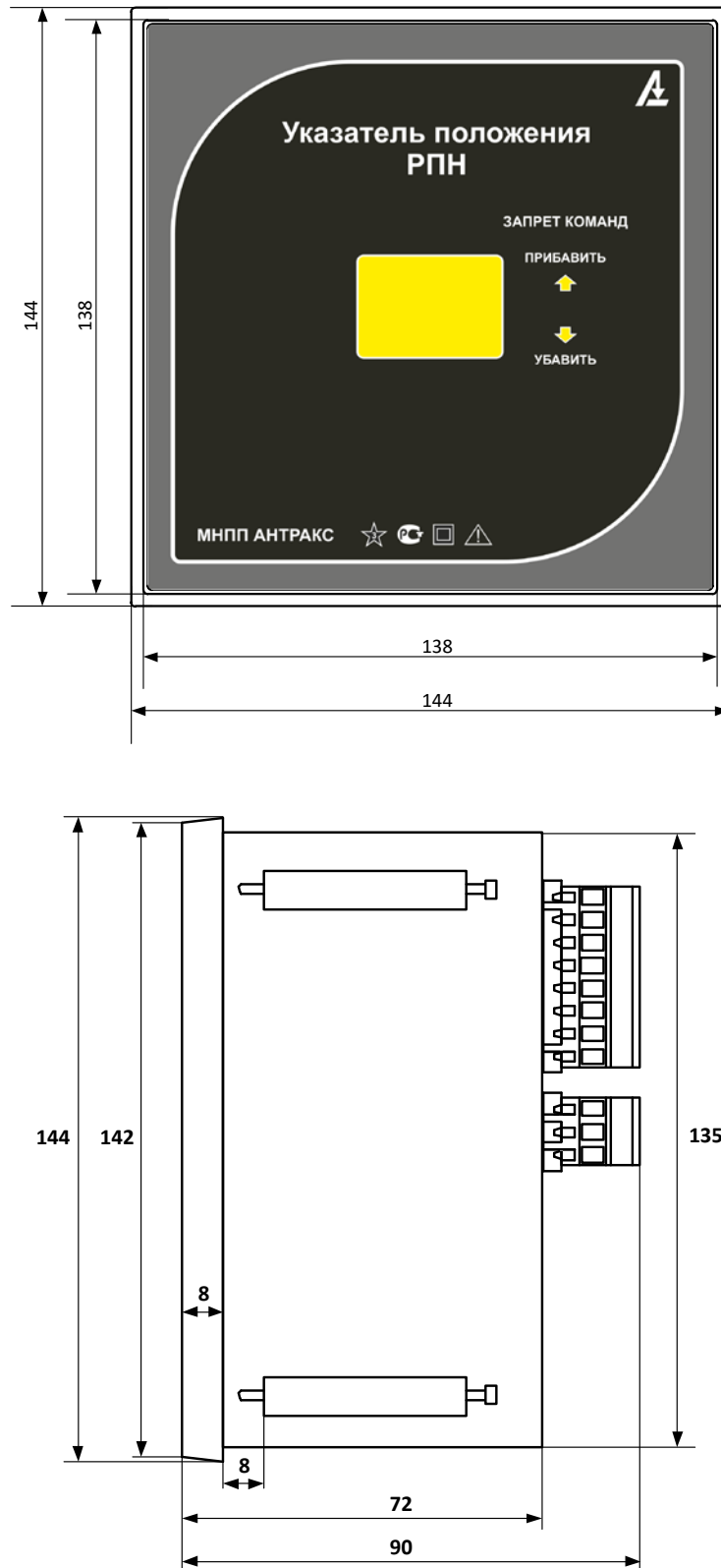
Рис. 1.1 Габаритные размеры щитового варианта указателя положения РПН УП 22-Б
