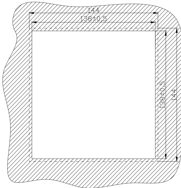
Рис. 2.1 Размеры вырубного окна в щите для установки щитового варианта указателя положения УП 22-Б
