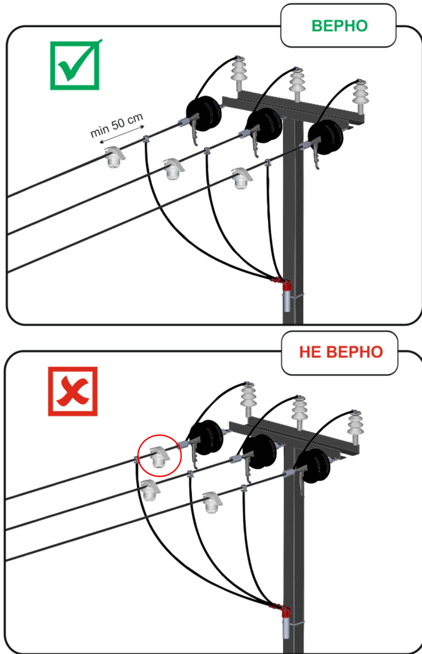
Рисунок 6 – Пример установки комплекта индикаторов ИКЗ-В33
