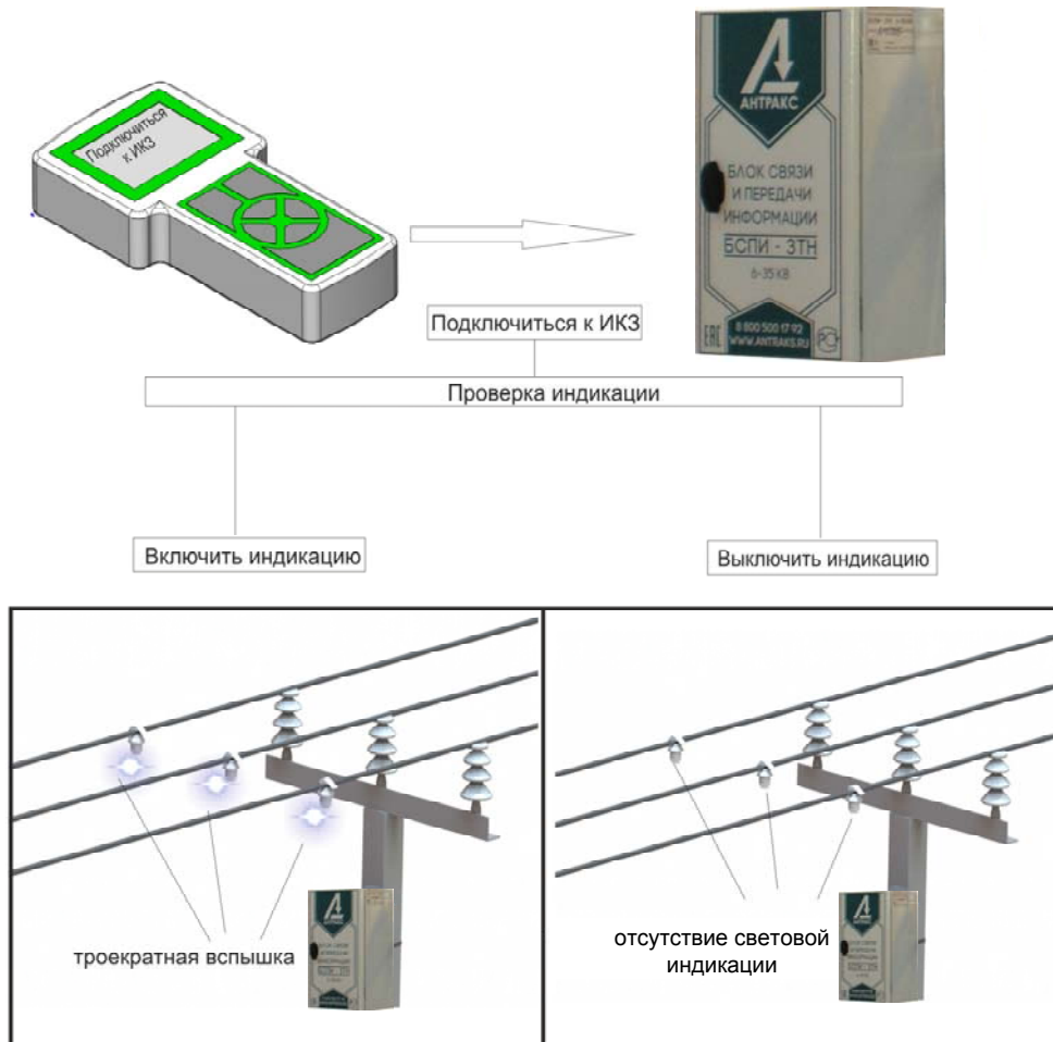
Рисунок 14 – Проверка работоспособности всего комплекта индикаторов ИКЗ-В33-ТНЗ
