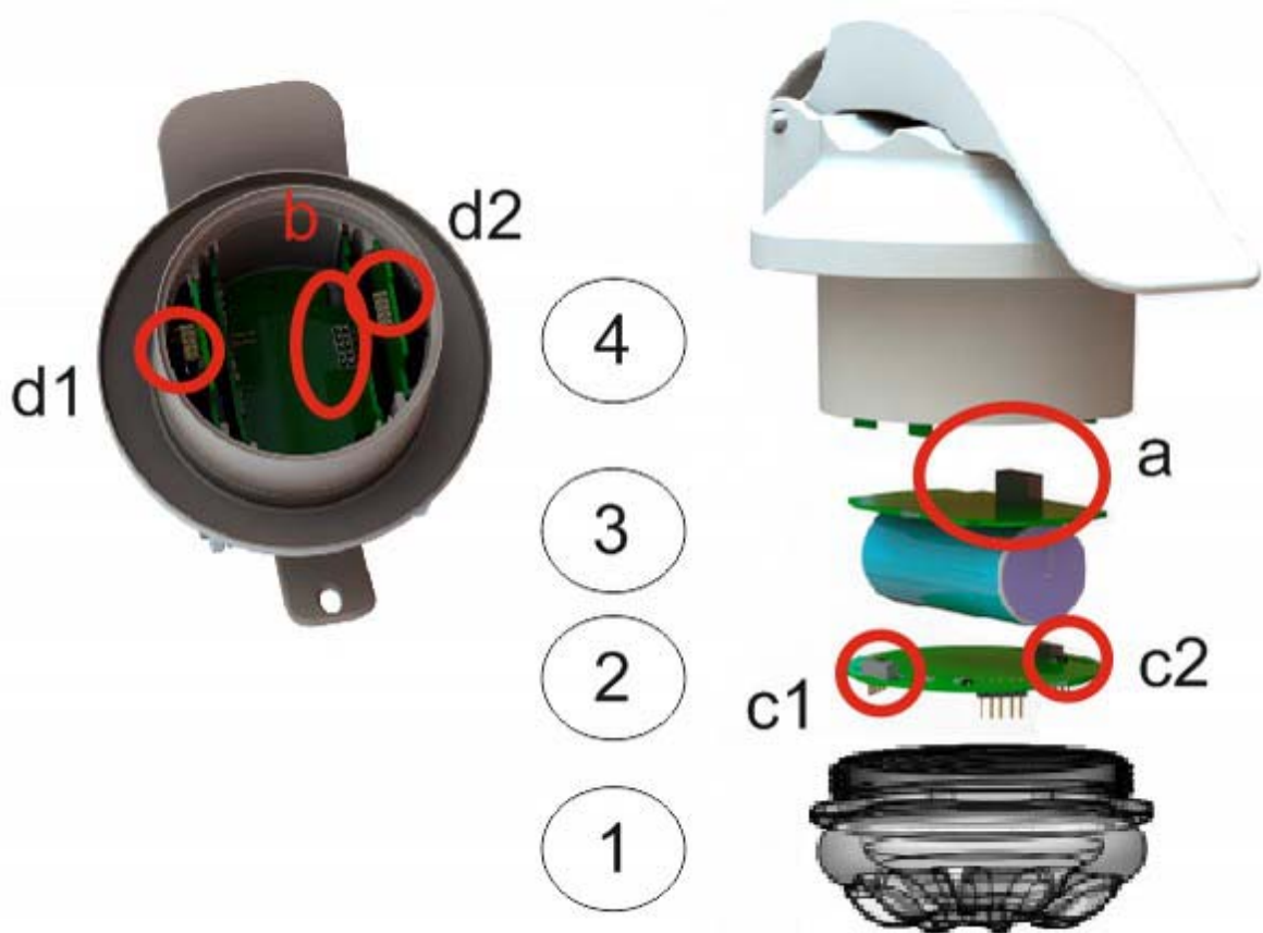
Рисунок 16 – Схема замены батарейного блока в индикаторе ИКЗ-В33
