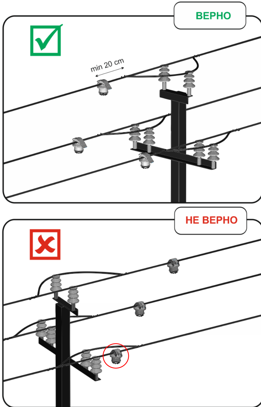
Рисунок 7 – Пример установки комплекта индикаторов ИКЗ-В33
