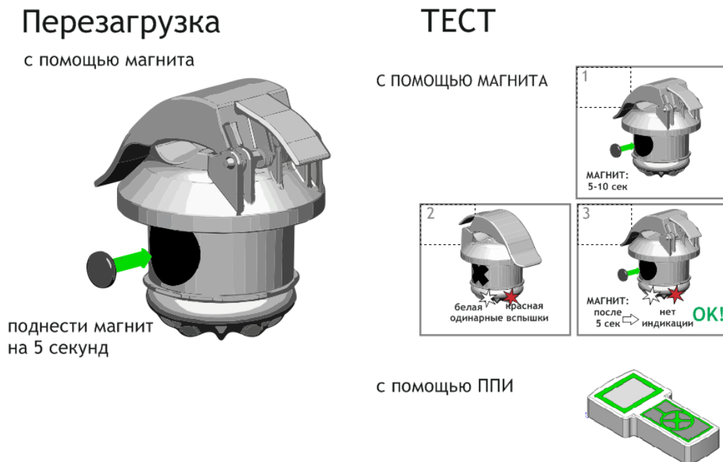
Рисунок 15 – Техническое обслуживание
