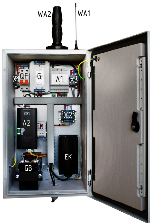
Рисунок 4.1 – Общий вид БСПИ-3ТН
