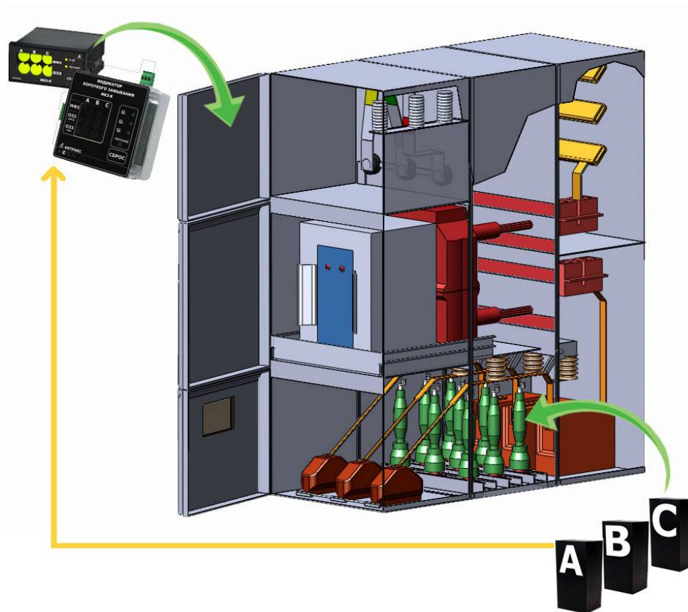
Рис. 3. Установка индикатора в ячейке КРУ.
