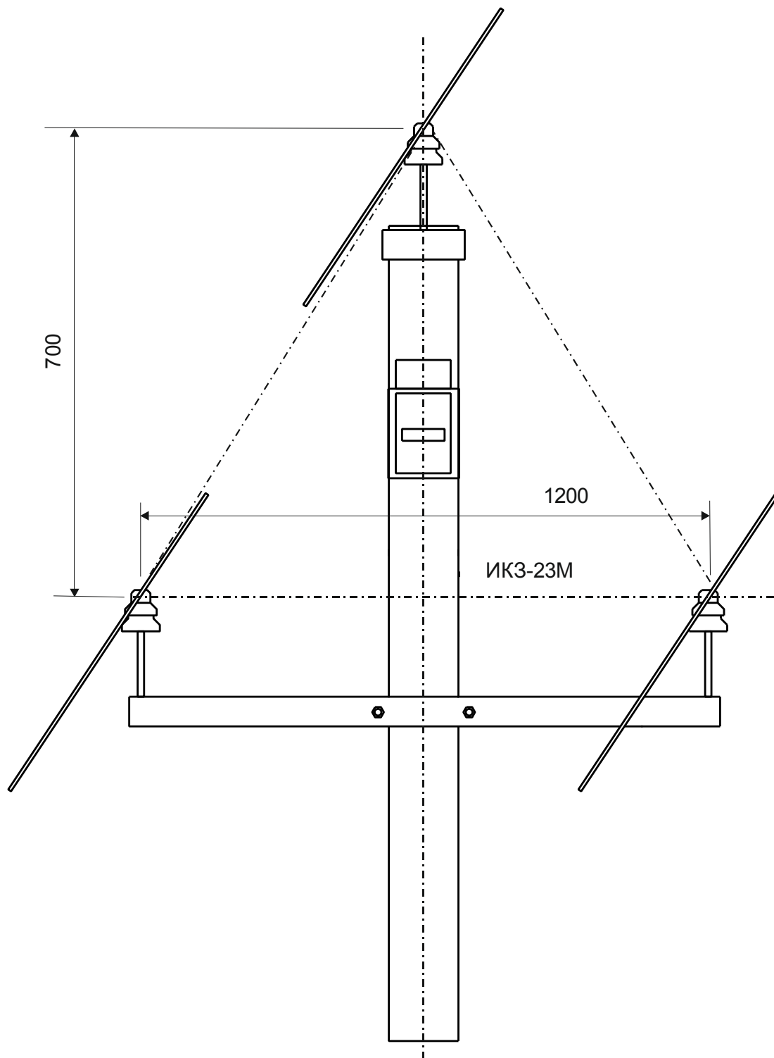
Рис. 2.2 Установка индикатора ИКЗ-23М на железобетонной опоре.
