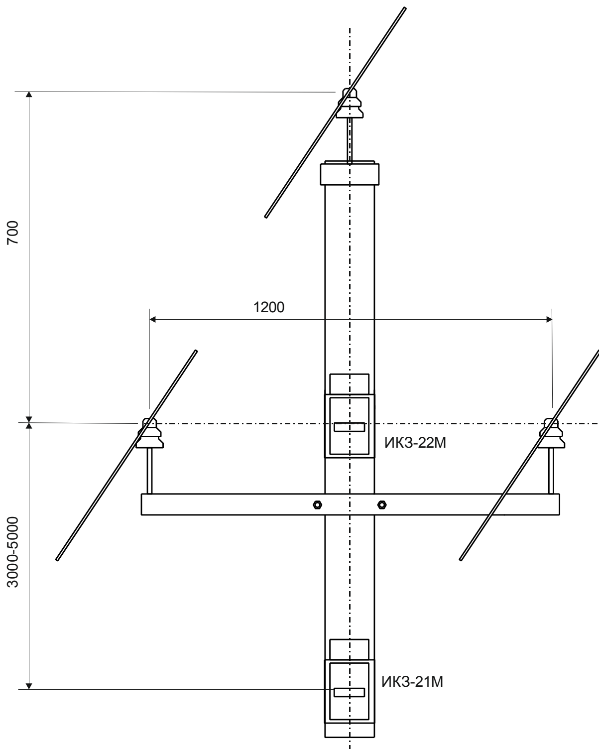
Рис. 2.1 Установка индикаторов ИКЗ-21М, ИКЗ-22М на железобетонной опоре.
