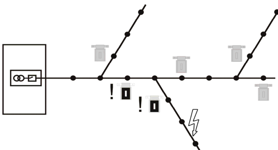
Рис 3 Установка индикаторов на линии с длинным стволом и длинными ответвлениями
