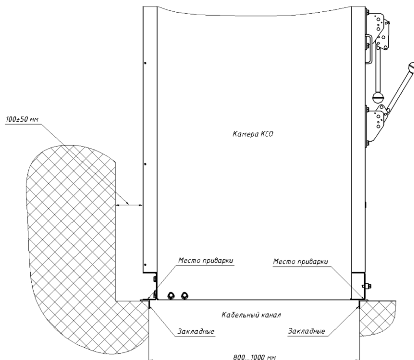
Рисунок 1. Установка камер КСО на закладные
