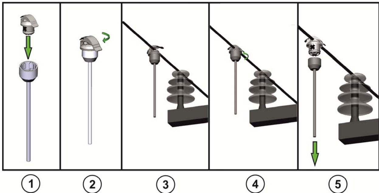
Рисунок 16 – Порядок установки индикатора ИКЗ-В31 без отключения подачи напряжения
