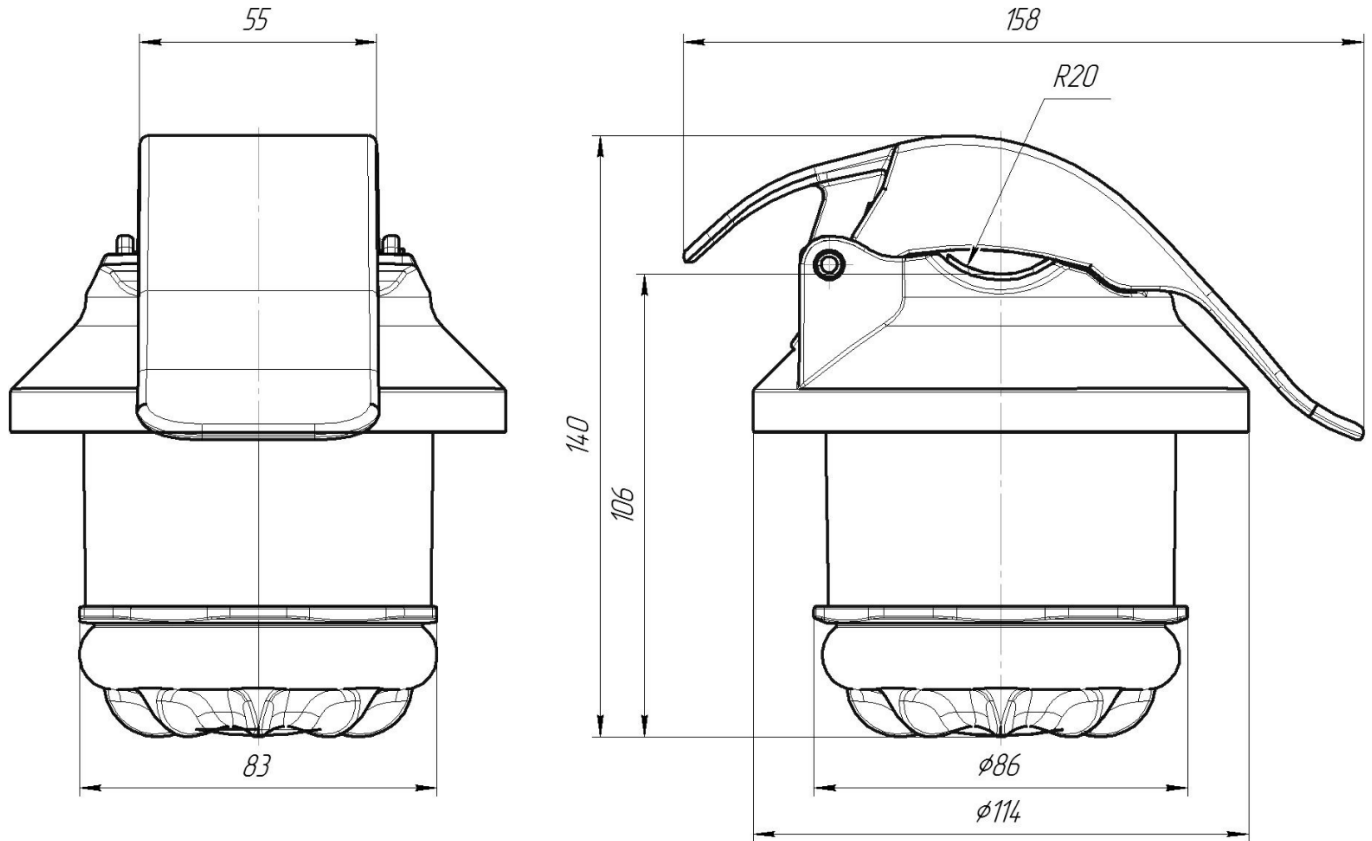
Рисунок 1.1 – Габаритные размеры ИКЗ-В3
